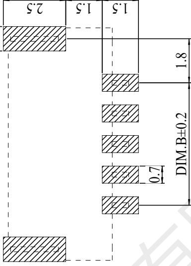
印制线路板
