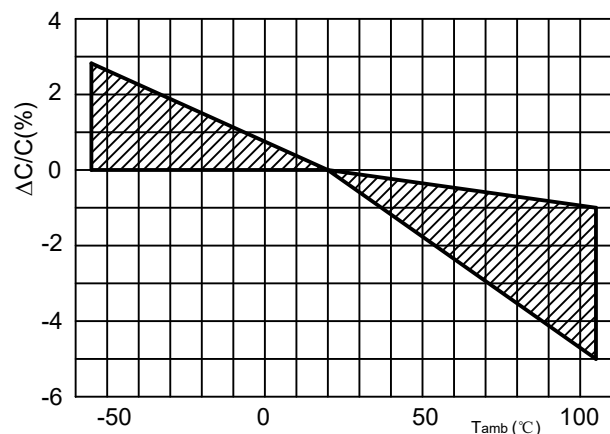
容量随温度变化曲线 (典型值)
