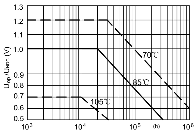
预期寿命曲线 (典型值)
