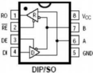
图1封装图
