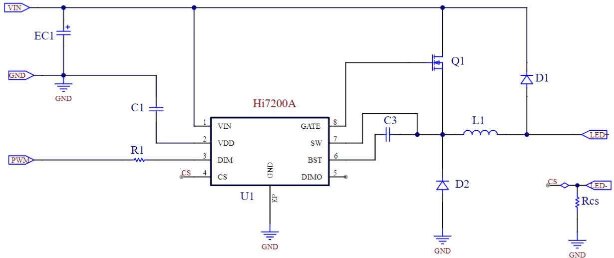
图 7.1 典型应用电路（不切光应用）
