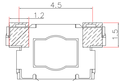
PCB板焊盘尺寸
