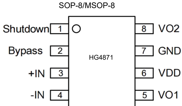
图 1. HG4871 的管脚定义图
