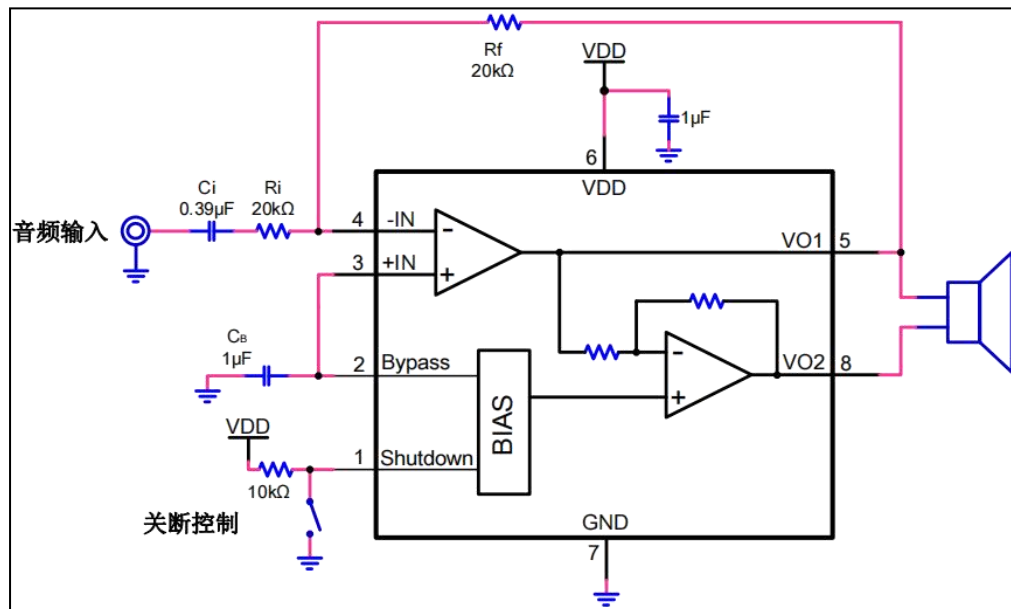
图 2. HG4871 单端输入模式电路图
