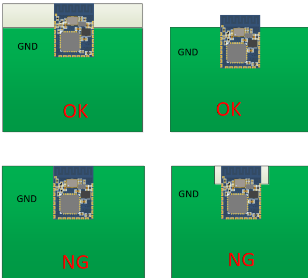
图 5-2 模块的摆放布局建议
