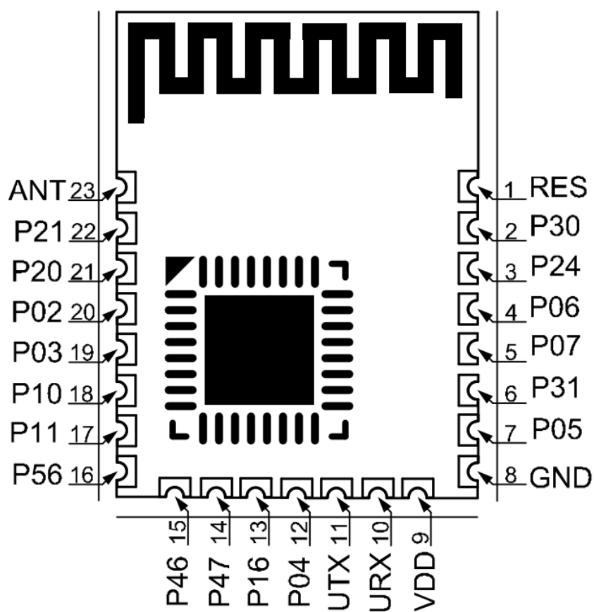
图 3-1 正面图
