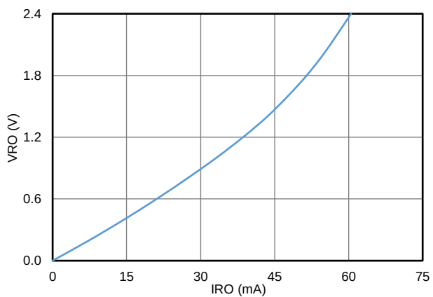
Fig. 9.4. 5V 供电下 RO 输出能力 (输出低电平)
