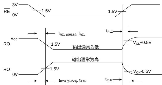
Fig. B4. 接收器使能和禁用时间
