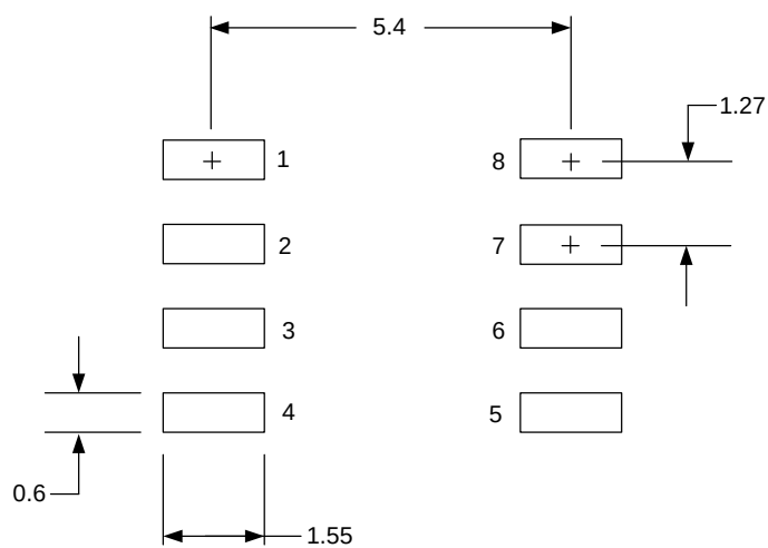
Fig. D1. SOP-8L(150mil)焊盘细节图 (所有尺寸单位为 mm)
