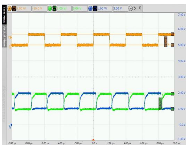
Fig. 9.9. 3.3V 供电下 500kbps 驱动波形 (485 总线负载 54Ω和 50pF, 室温)
