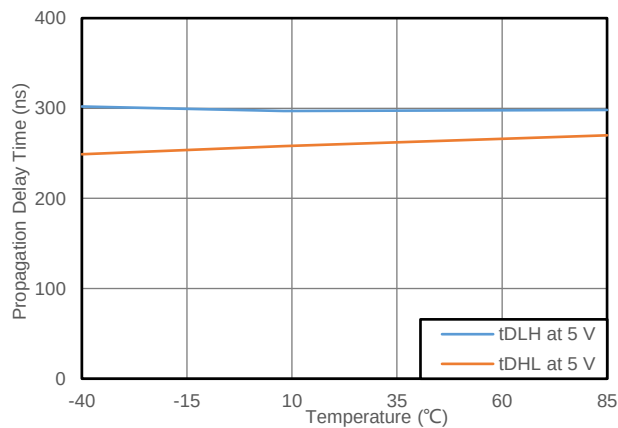
Fig. 9.6. 5V 驱动器传输延时
