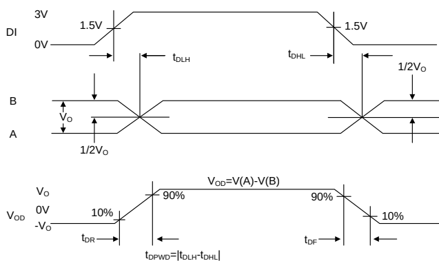
Fig. B2. 驱动器上升下降时间和传输延时
