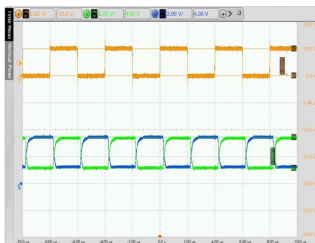
Fig. 9.10. 5V 供电下 500kbps 驱动波形 (485 总线负载 54Ω和 50pF, 室温)
