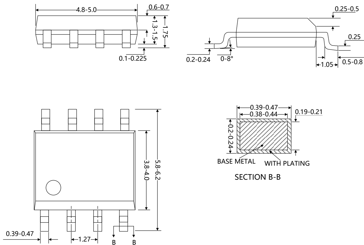
Fig. C1. SOP-8L(150mil) (所有尺寸单位为 mm)
