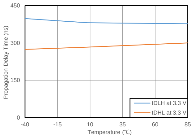
Fig. 9.5. 3.3V 驱动器传输延时
