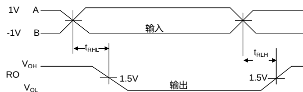
Fig. B3. 接收器上升下降时间和传输延时
