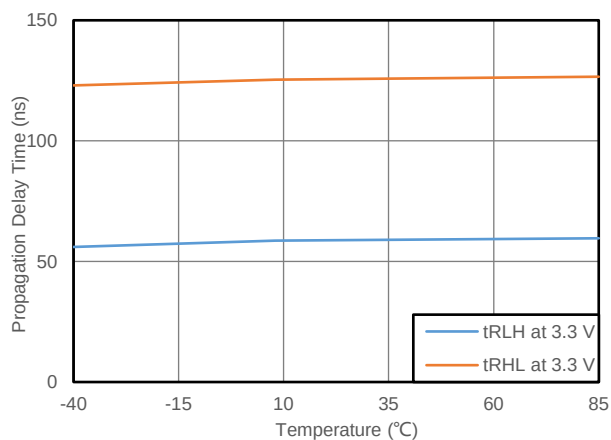
Fig. 9.7. 3.3V 接收器传输延时
