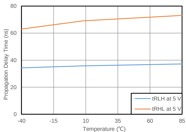
Fig. 9.8. 5V 接收器传输延时
