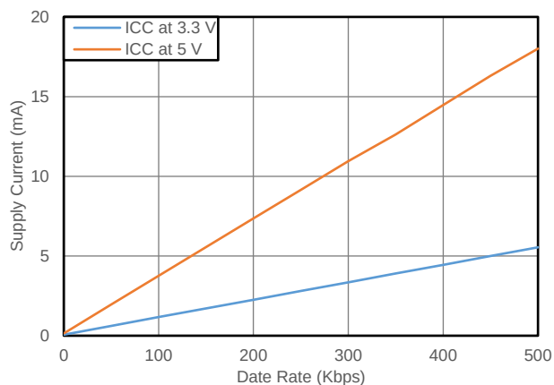
Fig. 9.1. 驱动电流和传输数据率的关系 (485 总线空载, 室温)
