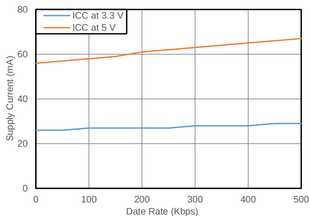
Fig. 9.2. 驱动电流和传输数据率的关系 (485 总线负载 54Ω和 50pF, 室温)
