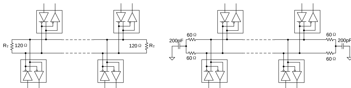
Fig. A2. 恰当的总线终端电阻匹配
