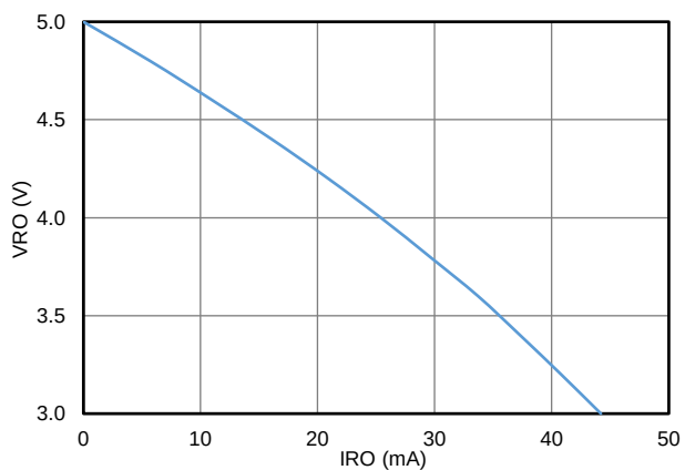
Fig. 9.3. 5V 供电下 RO 输出能力 (输出高电平)
