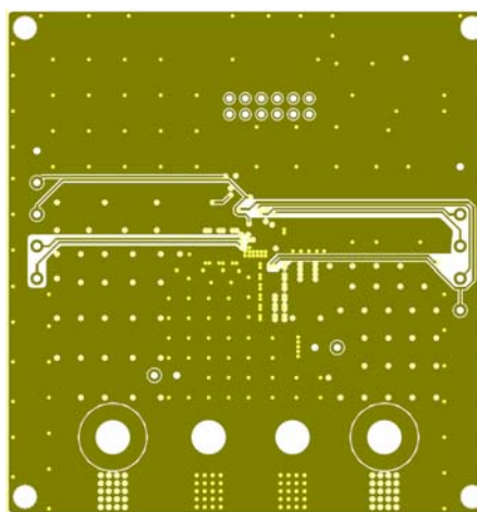
Figure 4— Inner Layer 2
