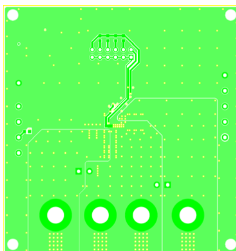
Figure 5—Bottom Layer
