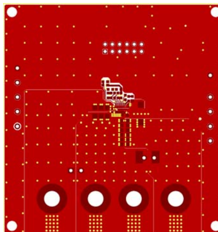
Figure 2—Top Layer
