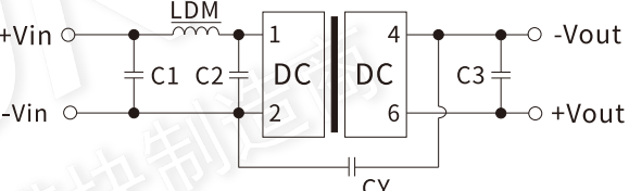
EMC推荐电路参数值 表(2)
