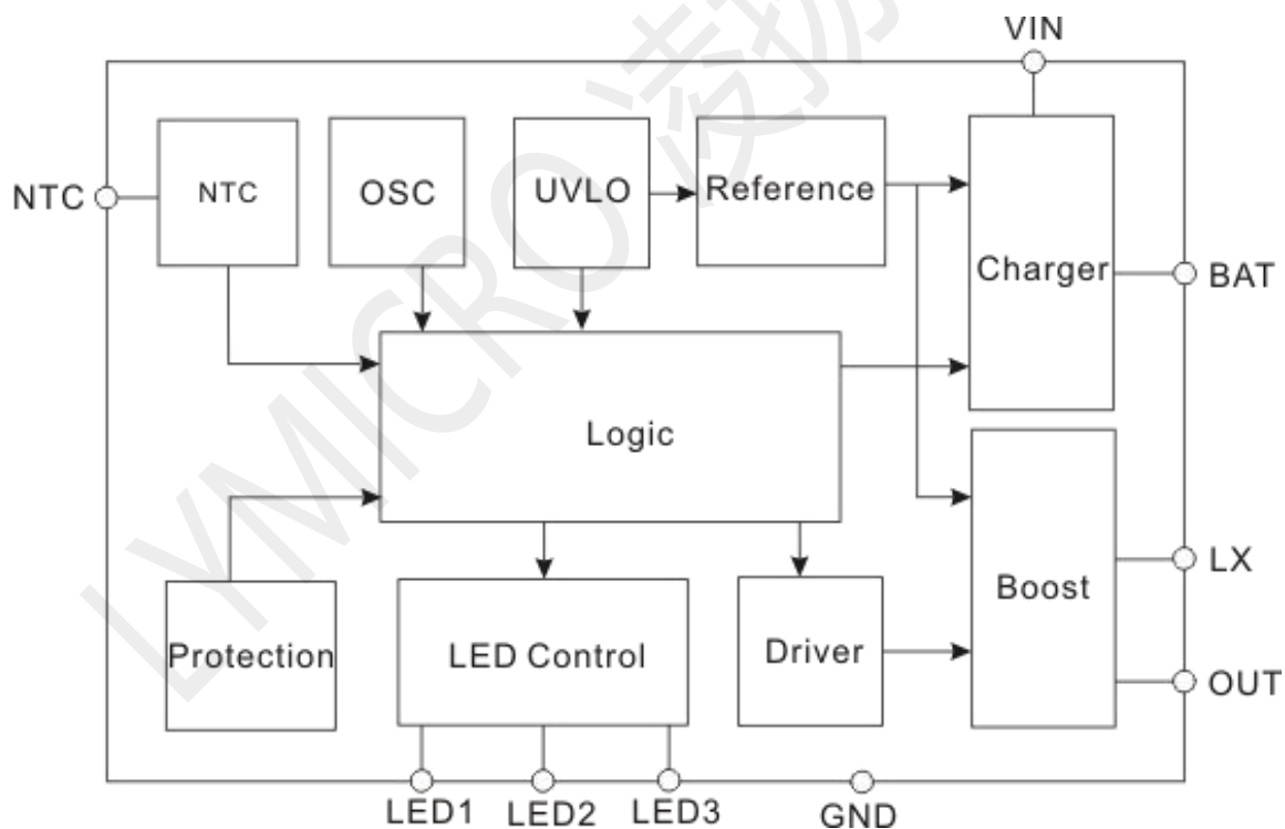
Fig3.功能框图
