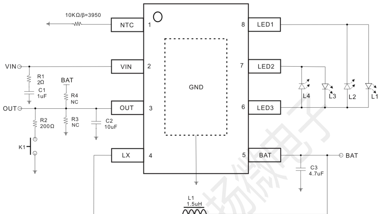
Fig1.LY6394T 典型应用电路
