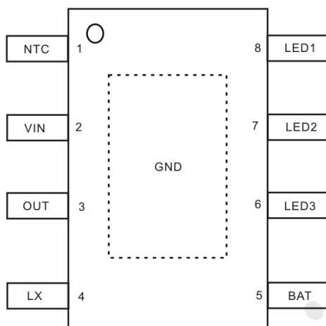
Fig4.管脚示意图
