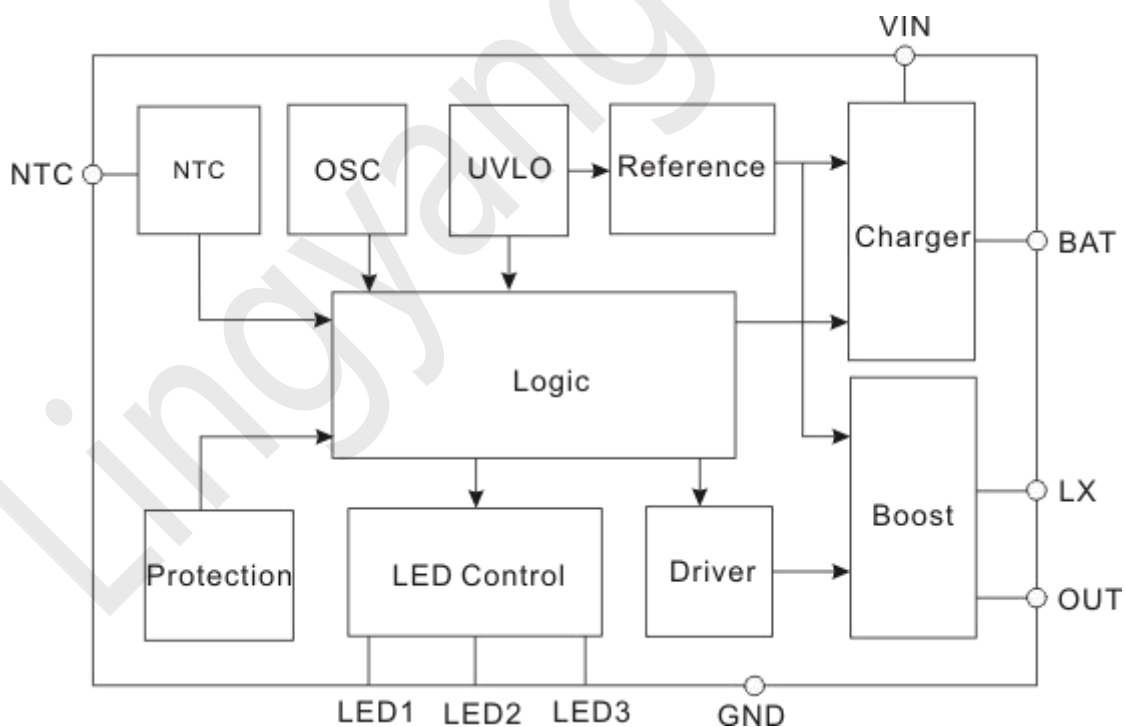
Fig3.功能框图
