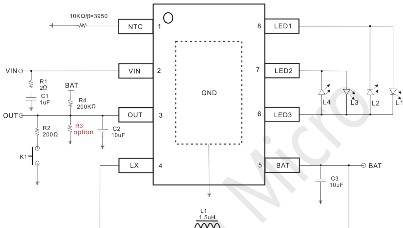
Fig1.LY6294T 典型应用电路
