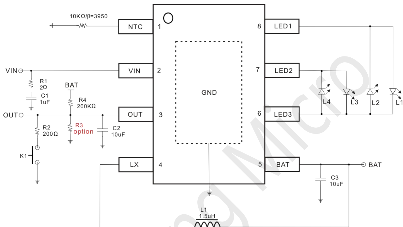
Fig5. 4 灯模式
