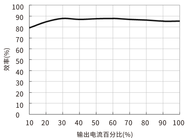
效率Vs输出负载(Vin=5V)
