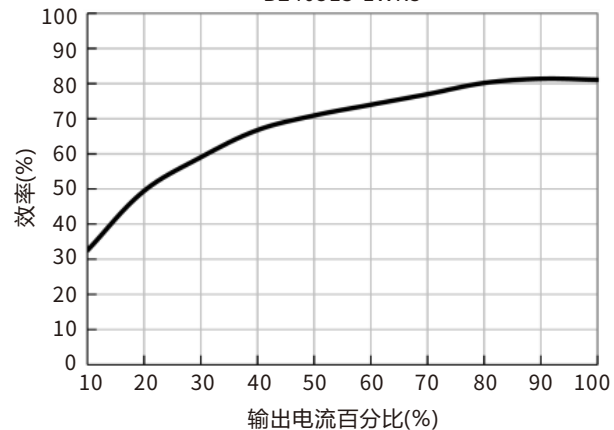
效率Vs输出负载(Vin=24V)
