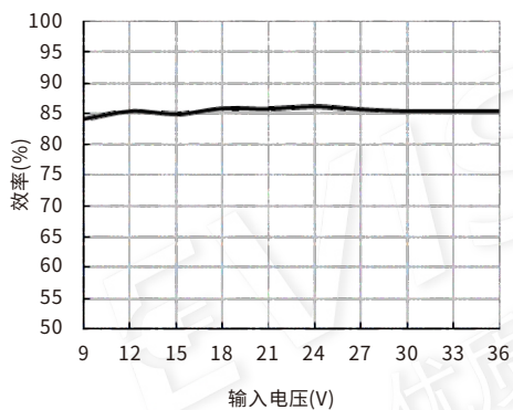
效率Vs输入电压(满载) URB2405ZP-10WR3
