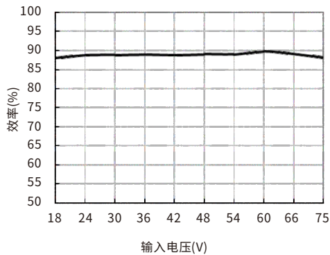
效率Vs输入电压(满载) URB4815ZP-10WR3
