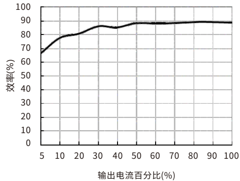
效率Vs输出负载(Vin=48V) URB4815ZP-10WR3
