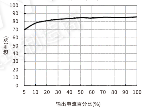
效率Vs输出负载(Vin=24V) URB2405ZP-10WR3
