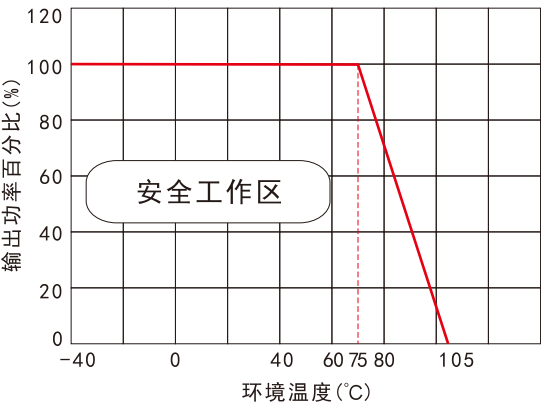
标称电压输入，12V、15V、24V输出 温度降额曲线图
