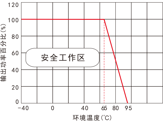
标称电压输入，3.3V、5V、6V输出 温度降额曲线图
