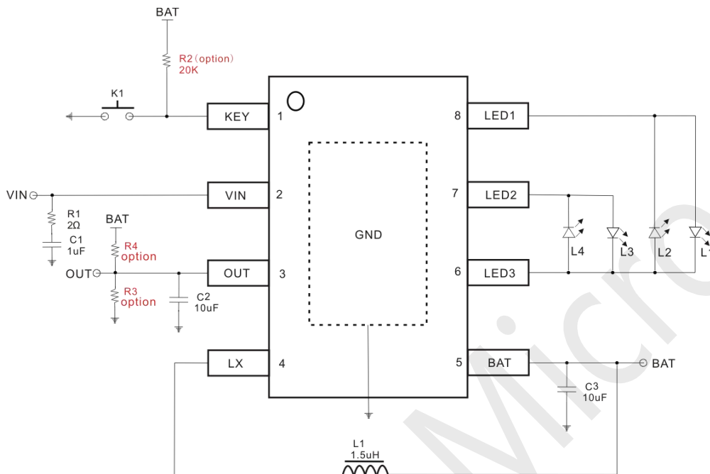
Fig1. LY6294 典型应用电路
