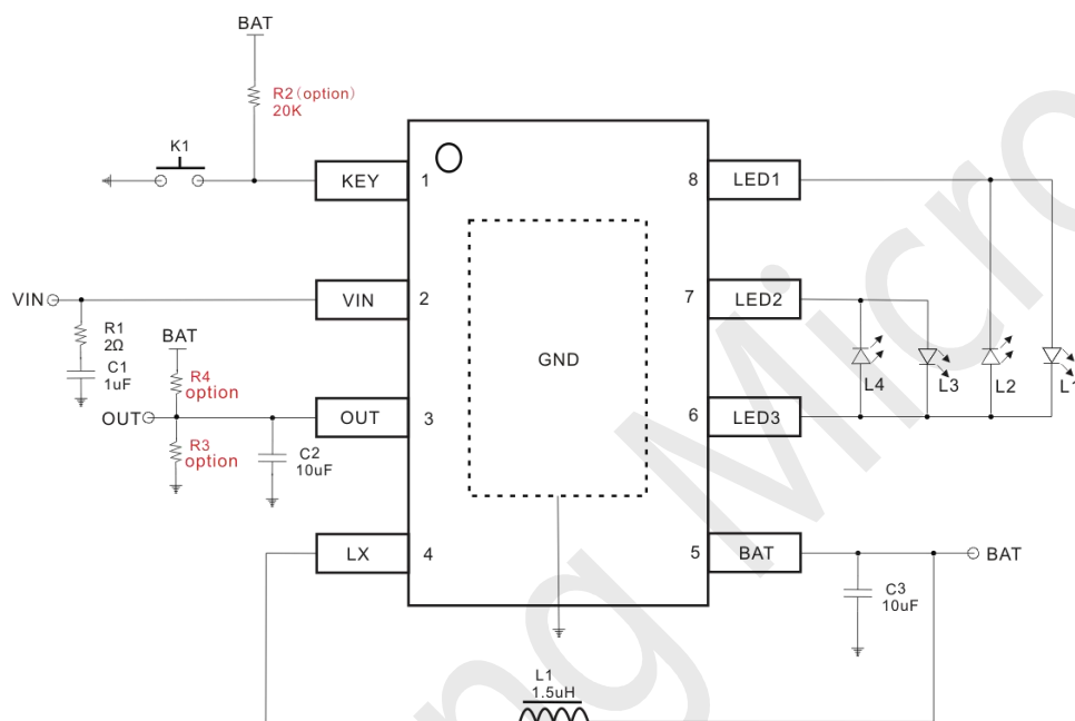
Fig4. 4 灯模式
