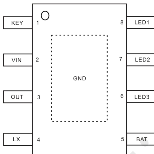
Fig3.管脚示意图
