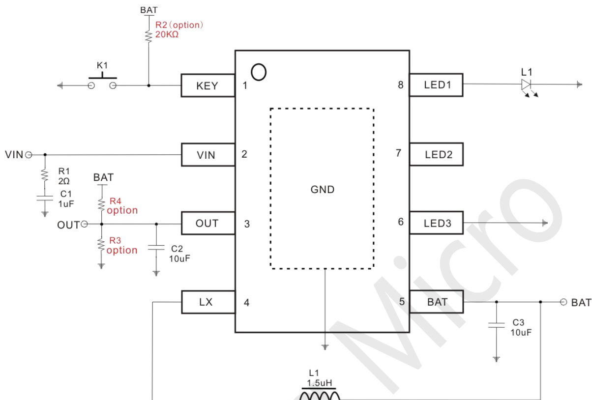
Fig8. 1 灯模式—2
