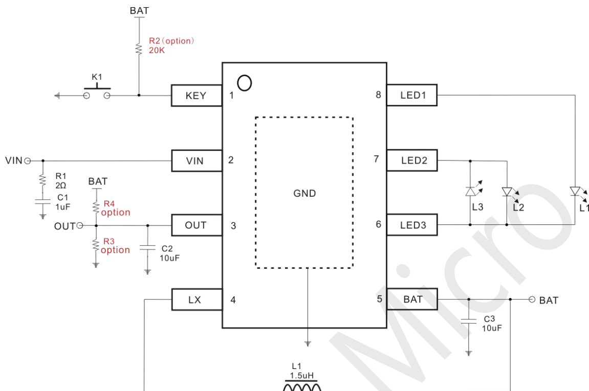
Fig5. 3 灯模式
