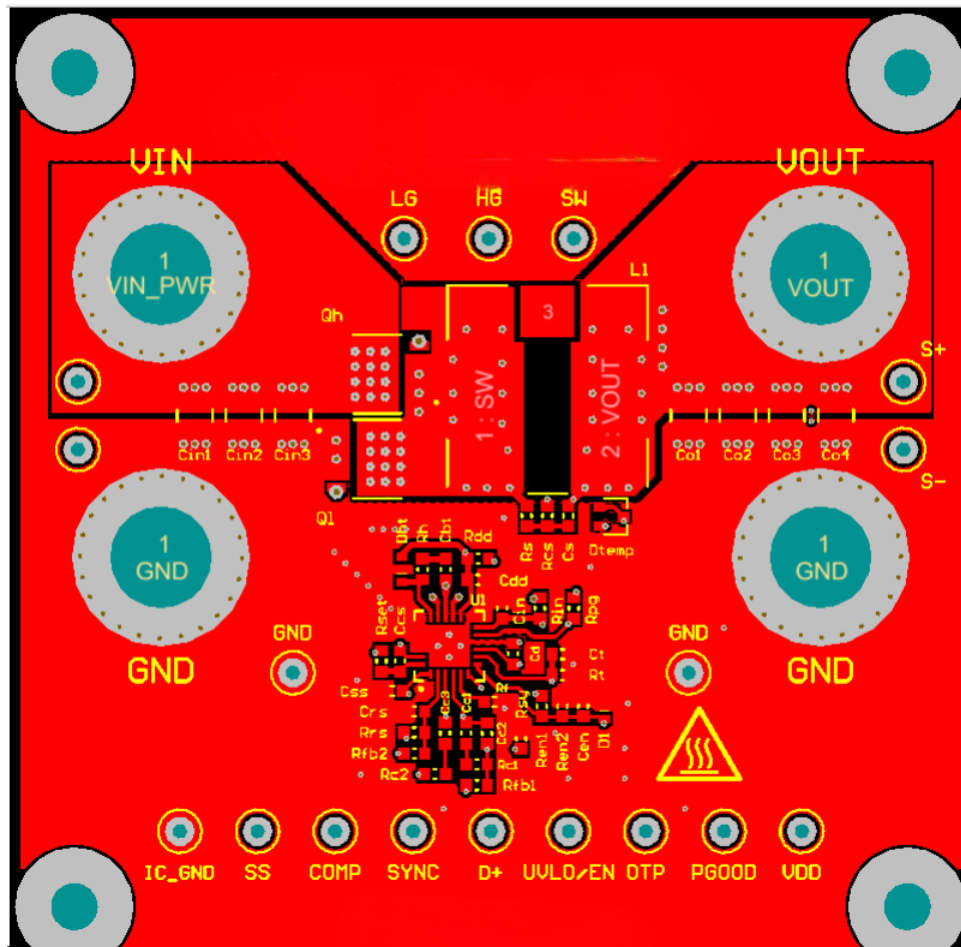
图 52. HT27403 PCB Layout
