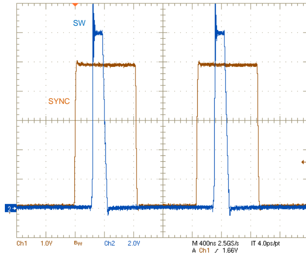
图 28. Typical 600-kHz SYNC Waveform
