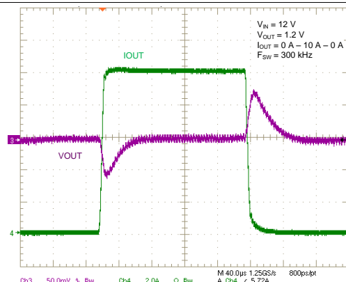
图 16. 10-A Step Load Transient Response, 2.5-A/ \mu s Slew Rate
