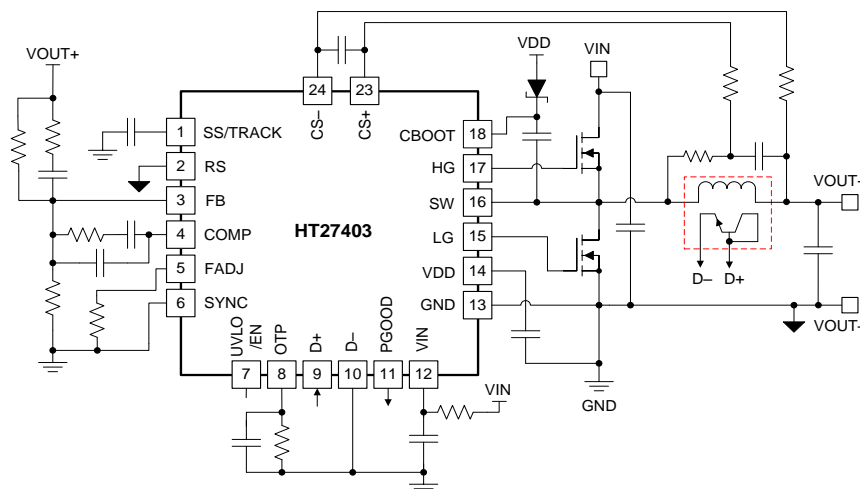
典型应用图
