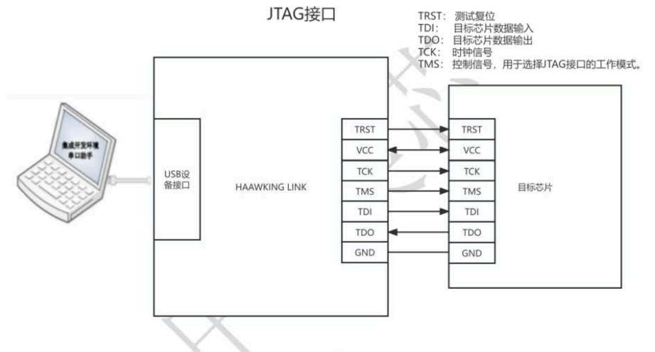
图 8-4. Haawking Link 连接示意图 (JTAG 接口)
