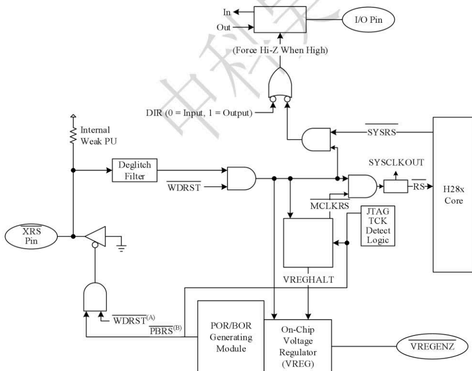
图 3-4 VREG+POR+BOR+复位信号连接
