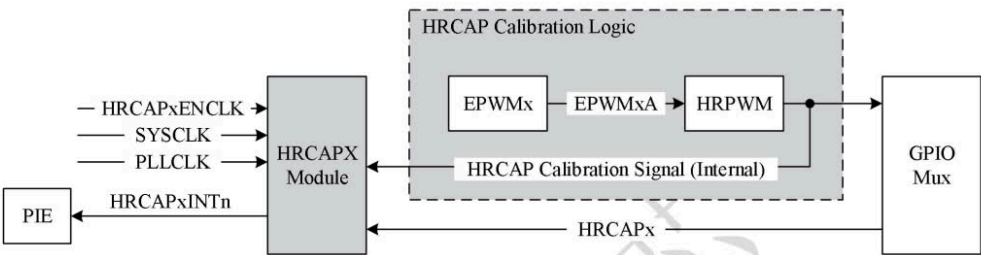
图 4-17 HRCAP 模块结构图
