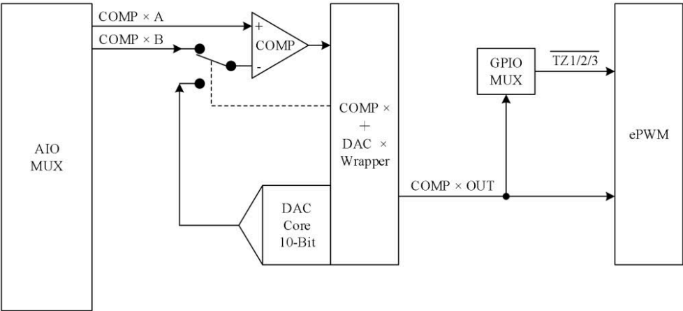
图 4-9 比较器模块结构框图
