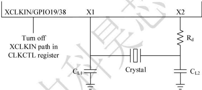
图 3-5 使用片上晶体振荡器
