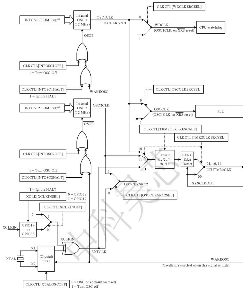
图 3-4 时钟树
