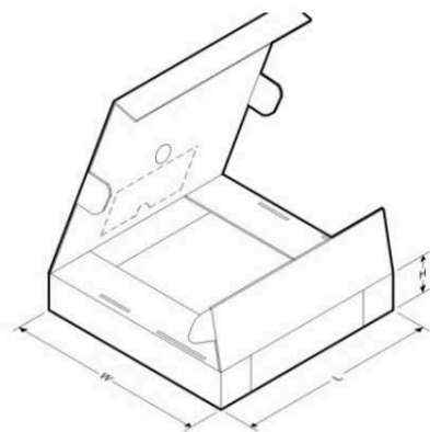
包装盒尺寸
