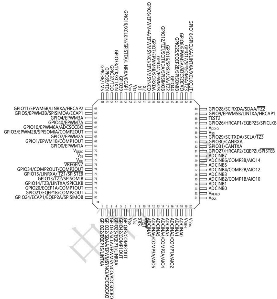
图 2-1 DSC28035 80 引脚 PN LQFP (顶视图)
