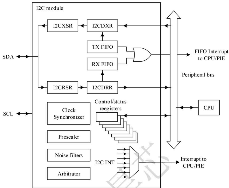
图 4-13 I2C 模块结构图
