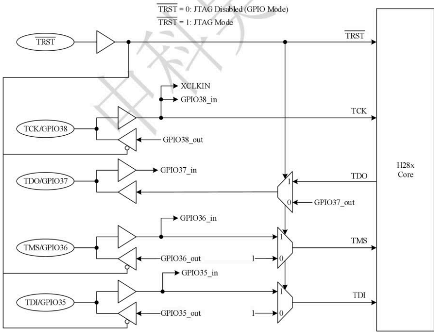
图 4-19 JTAG 端口多路复用示意图
