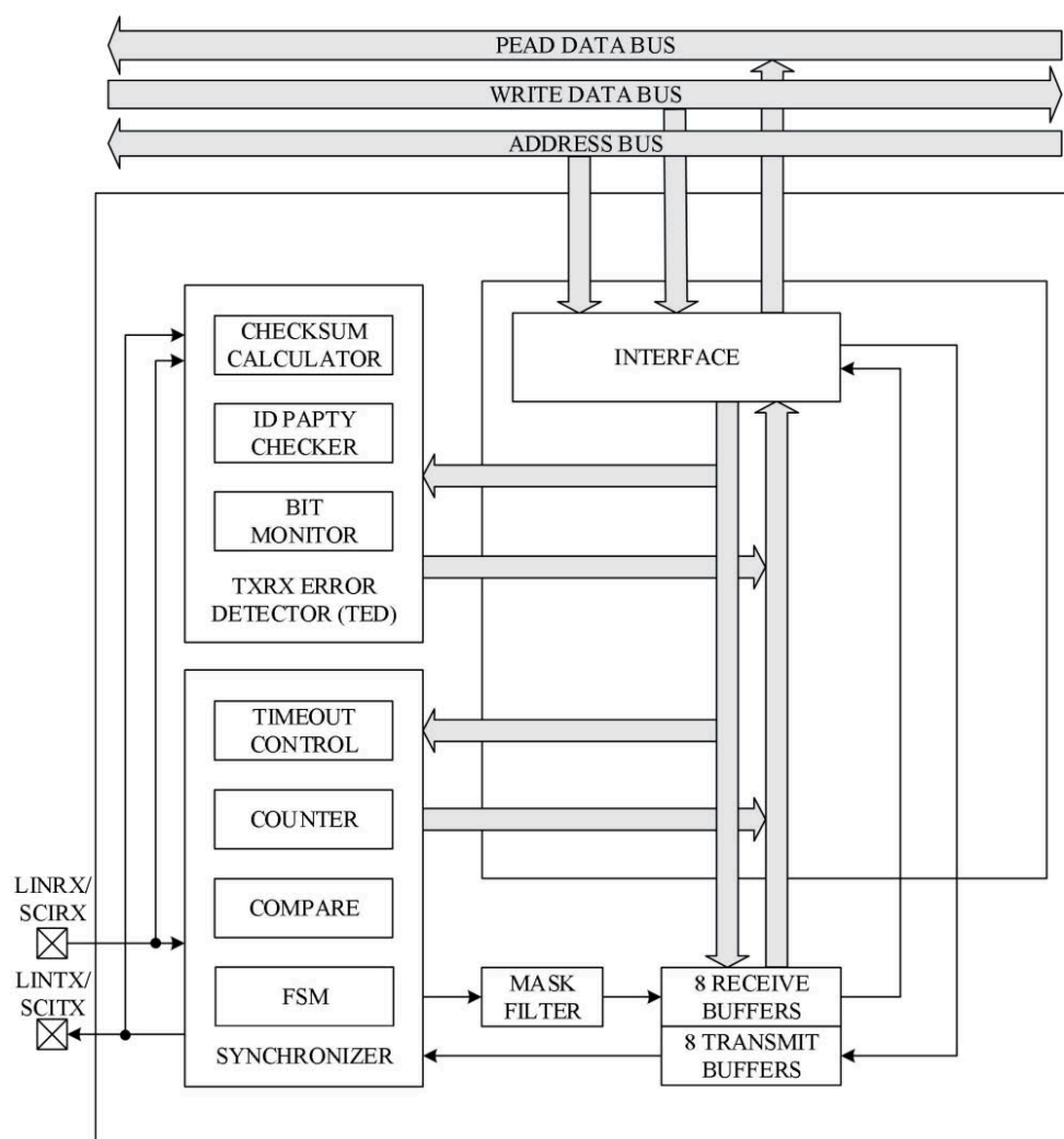
图 4-11 LIN 模块的结构图
