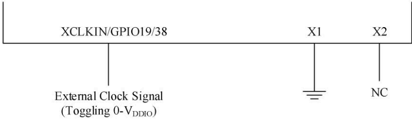
图 3-6 使用 3.3v 片外晶体振荡器
