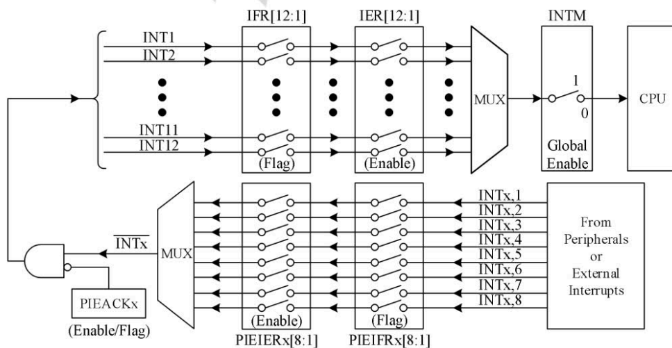
图 3-3 PIE 中断映射示意图
