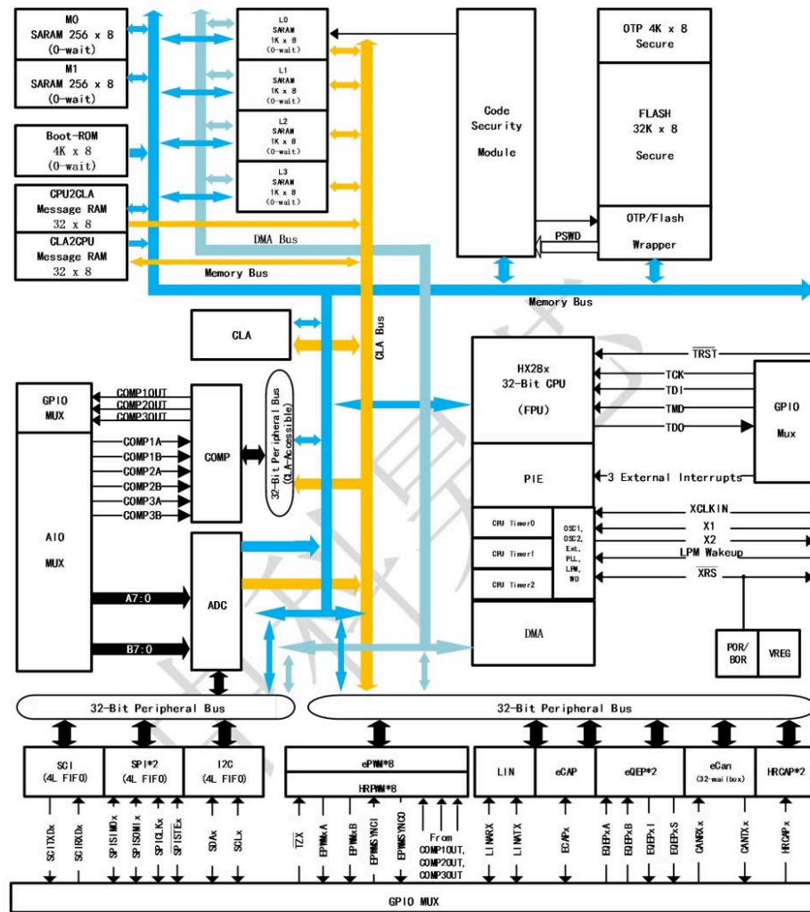
图 3-1 HXS320F28035 芯片架构图
