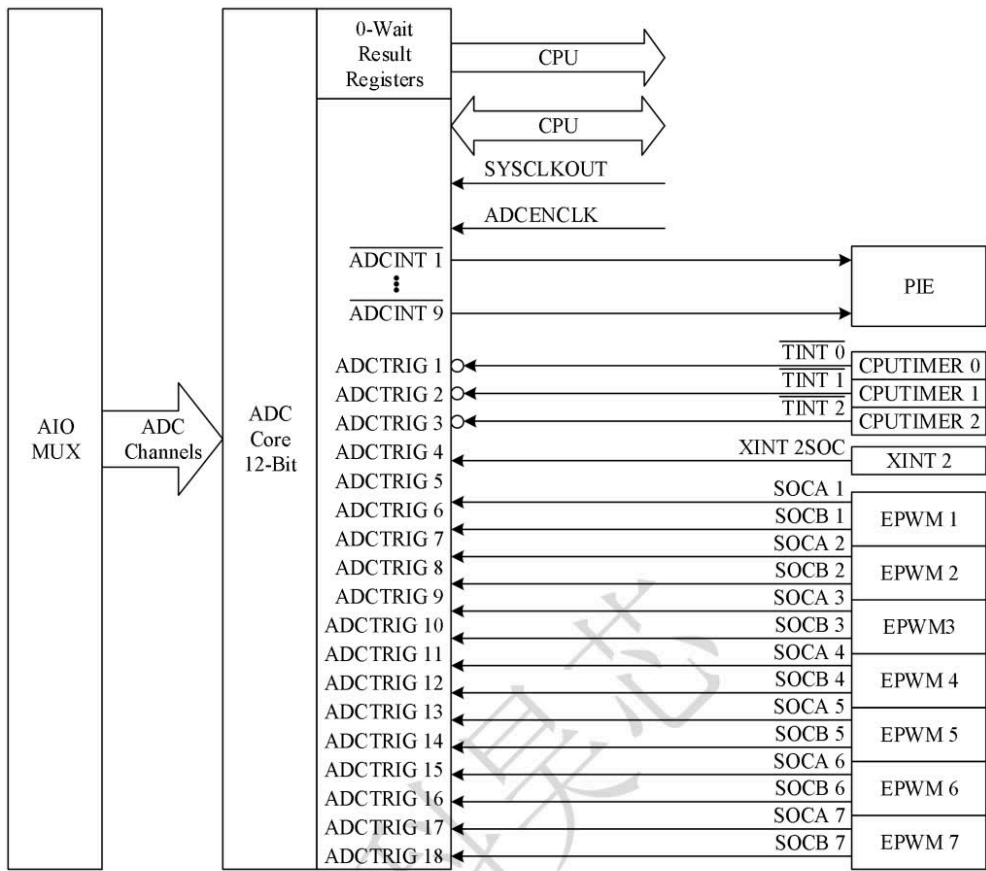
图 4-2 ADC 模块连接图
