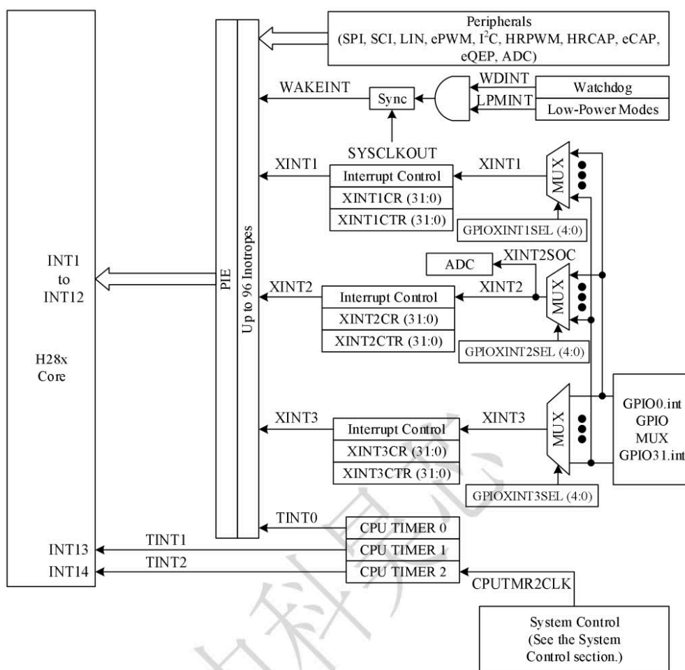
图 3-2 PIE 模块互联示意图
