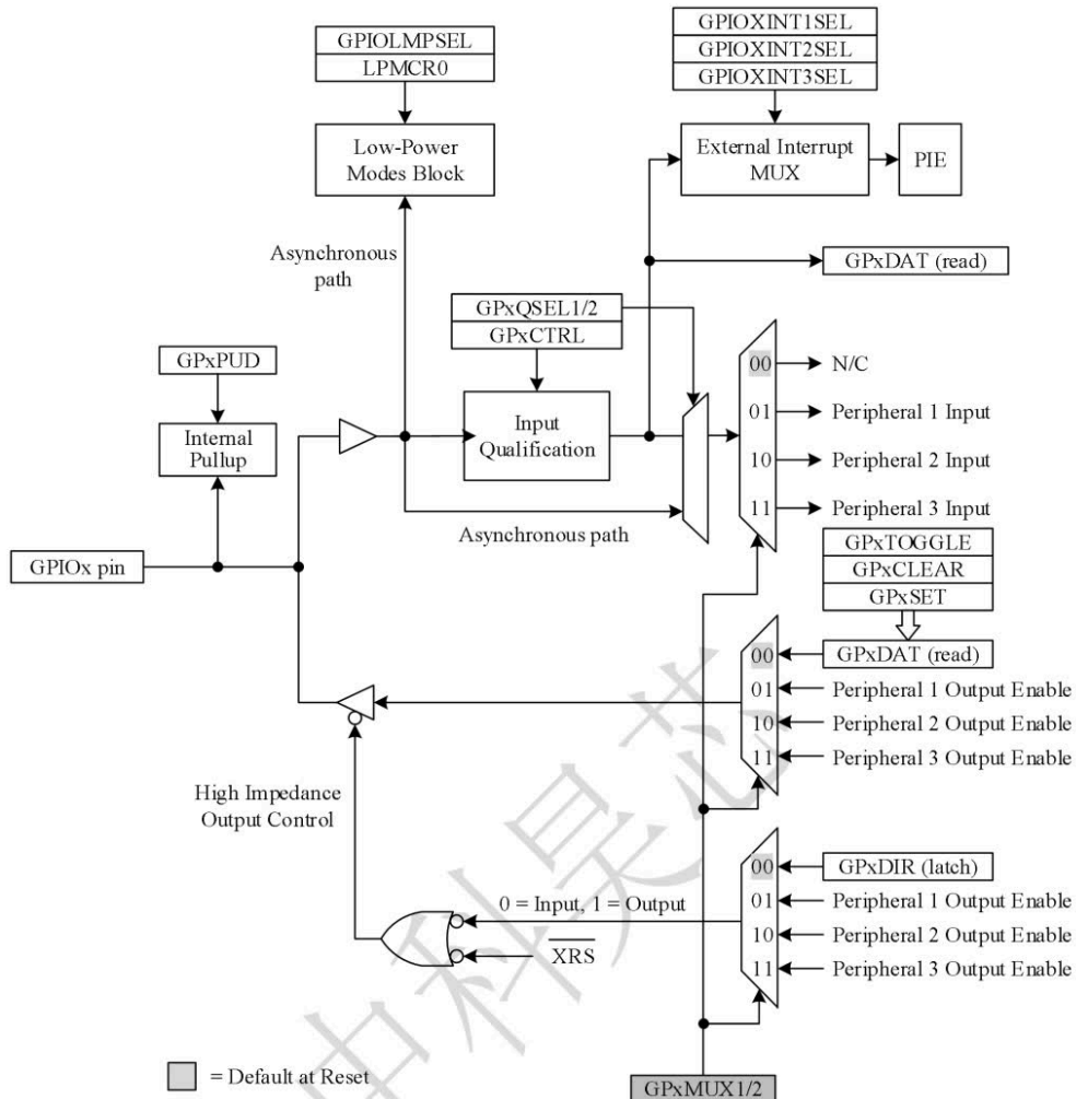
图 4-20 GPIO 复用模块连接示意图
