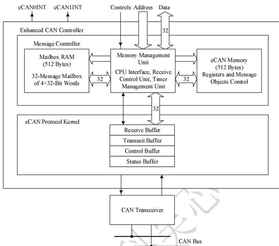
图 4-12 eCAN 模块的架构图和互联示意
