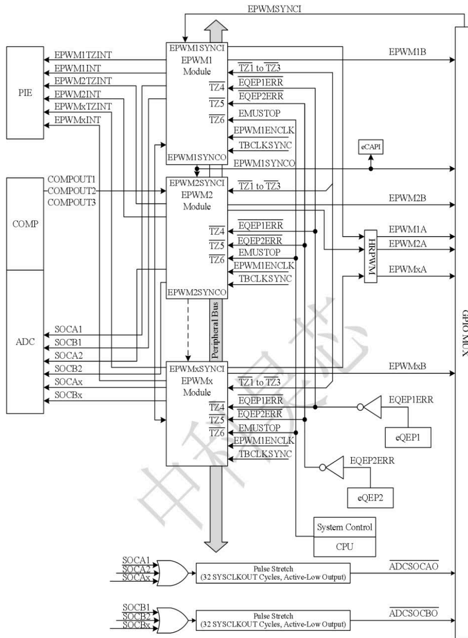
图 4-14 ePWM 模块结构图
