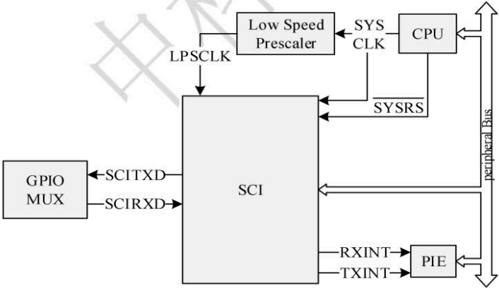
图 4-10 SCI 连接关系图
