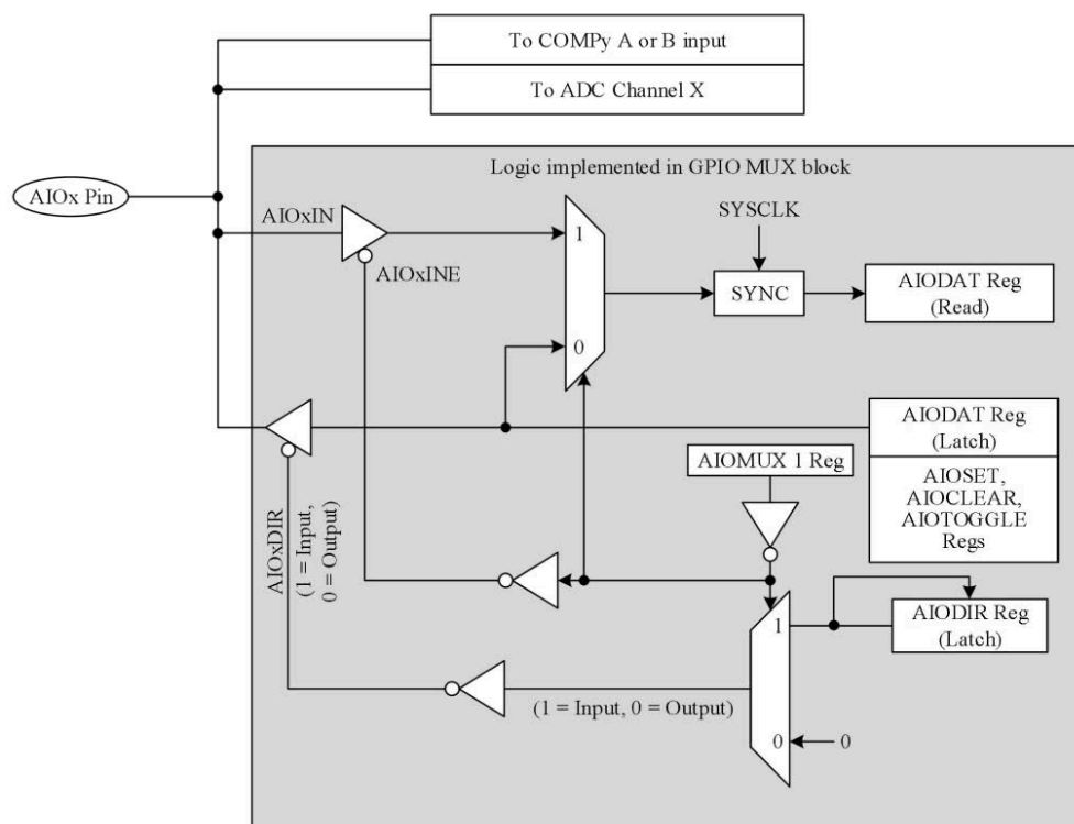
图 4-8 AIOx 引脚复用
