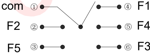
电路图
