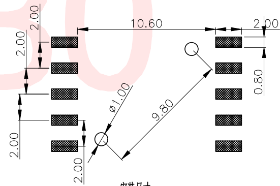
安装尺寸
