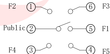
电路图
