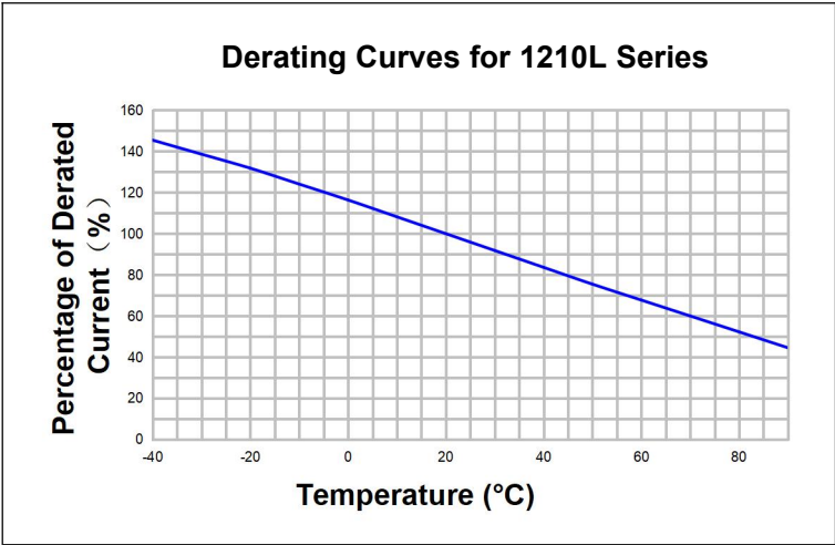
Thermal Derating Curve/环境温度与工作电流关系特性图
