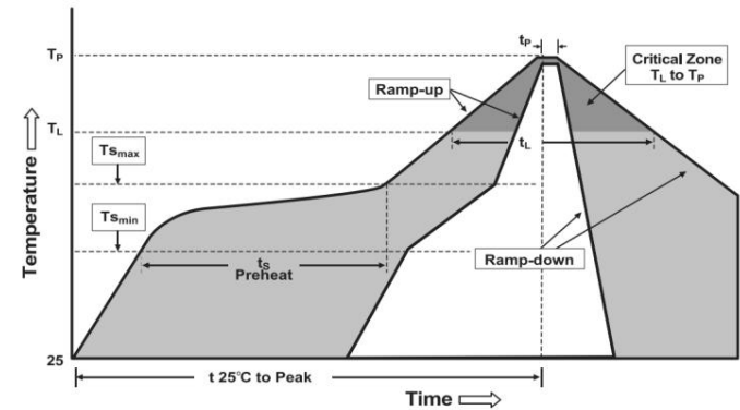
Soldering Parameters/焊接参数
