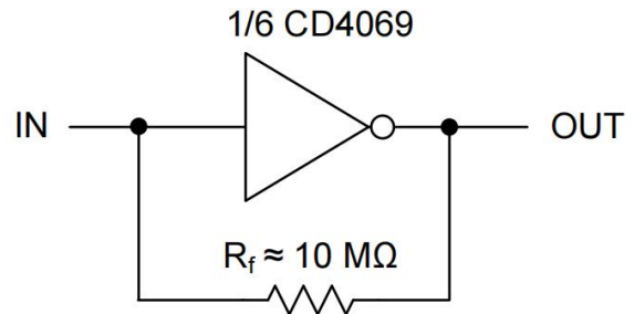
图 4 高输入阻抗放大器
