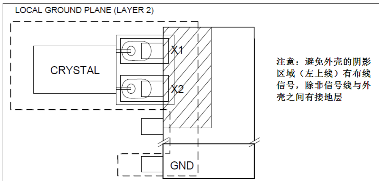
图2 晶振印刷电路板布局
