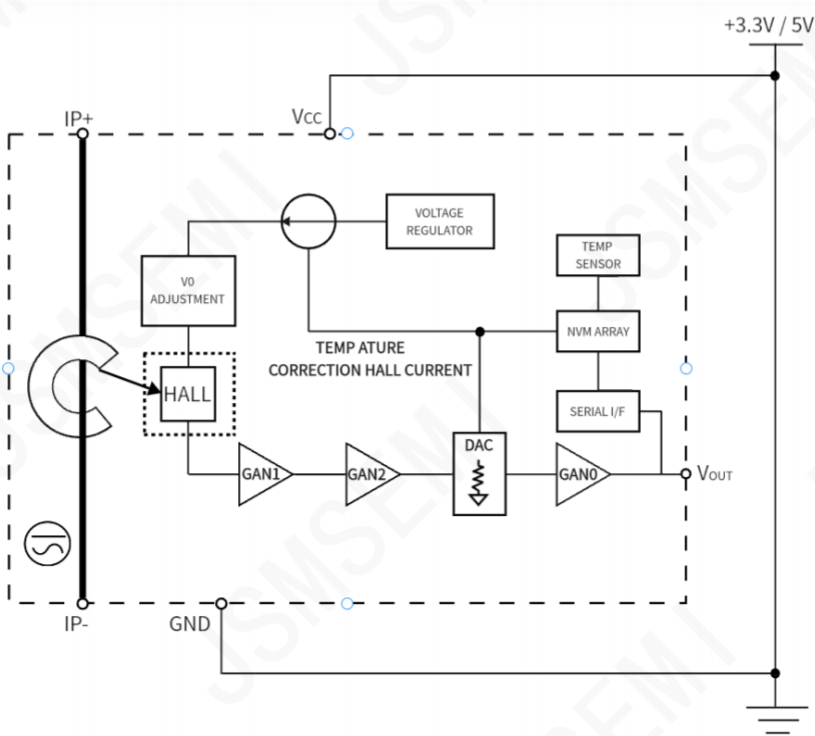
内部功能框图
