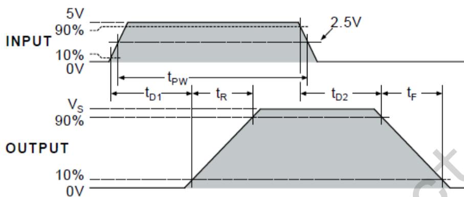
图 6-1 输入输出(同相)波形图
