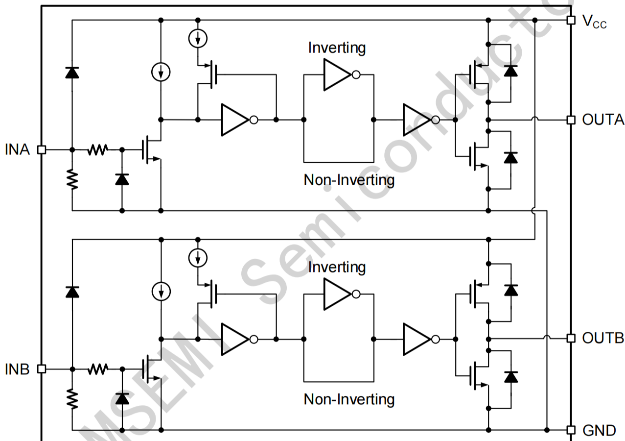
图 7-1 SID1127功能框图
