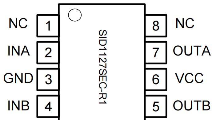
引脚描述
