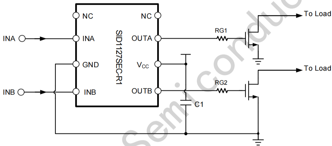
图 8-1 SID1127 典型应用电路图
