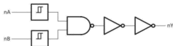
逻辑框图 (单路)
