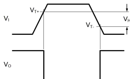
图 4 V_{T+} 、 V_{T-} 和 V_H 的定义
