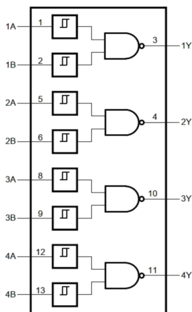
功能框图
