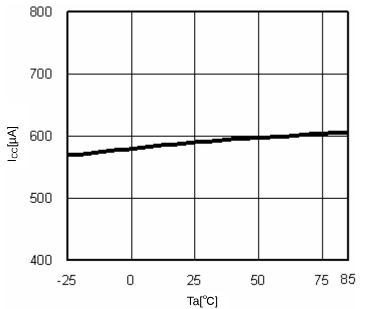
Fig.10 T_a-I_{CC}
