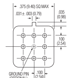
MGA/MGAD/MGADD Header
