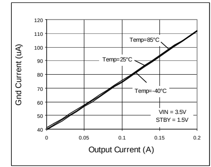
Fig. 39 IOUT - IGND
