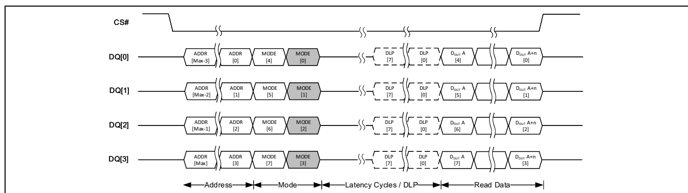
Figure 35 アドレスとモード入力のある QPI DDR 連続読み出しトランザクション (出力レイテンシ有り) [7]
