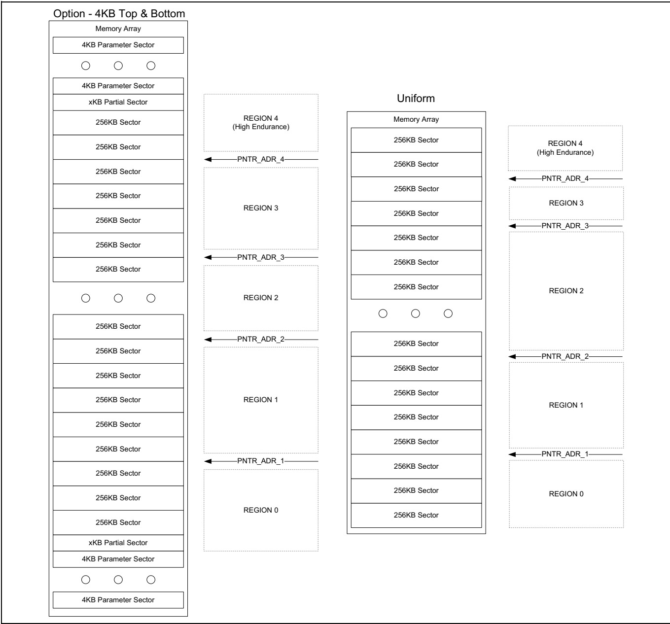
Figure 42 インフィニオン Endurance Flex アーキテクチャ概要 ( 続く )
