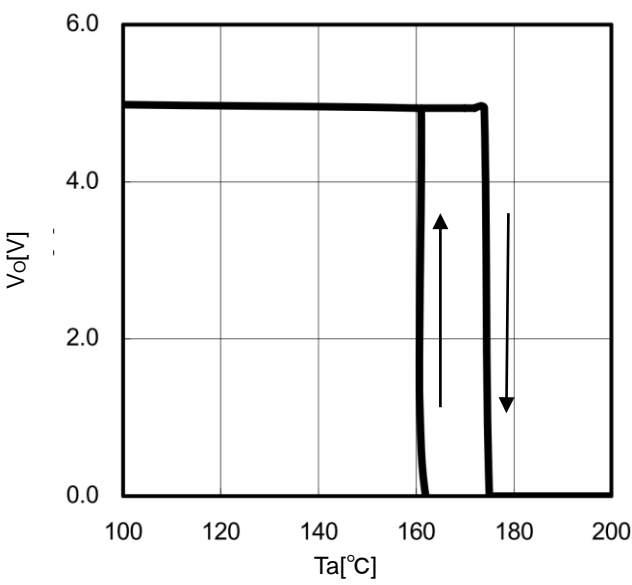
Fig.28 TSD (Io=0mA)
