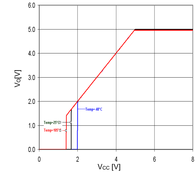
Fig.27 Vcc-Vo (Io=0mA)
