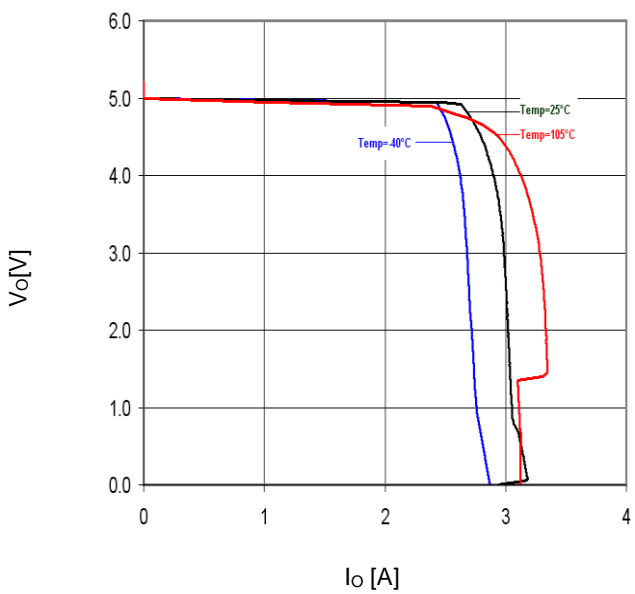
Fig.29 Io-Vo
