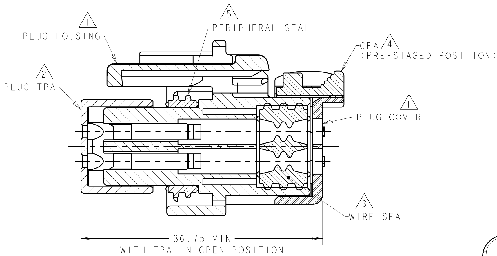
SECTION A-A
