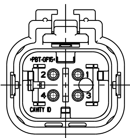
2320922-3 SCALE 2:1
