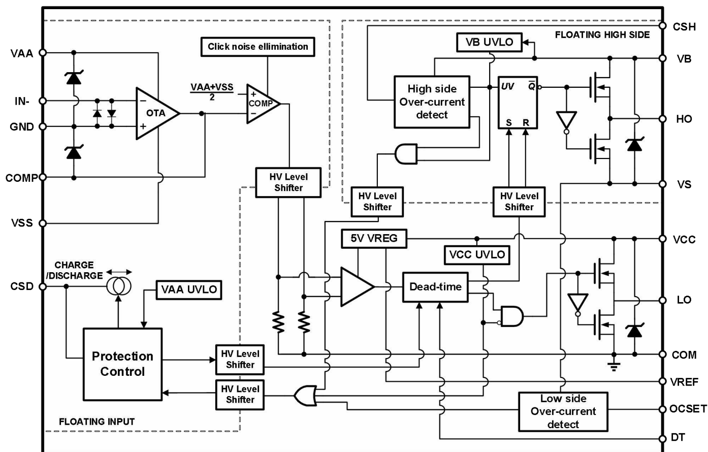
图7-1 全芯片功能框图
