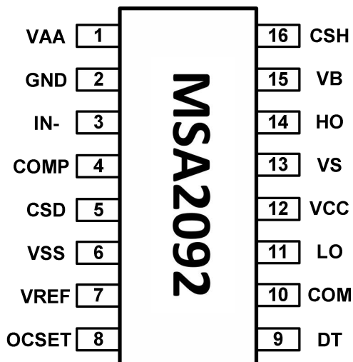
SOP-16 顶视图
