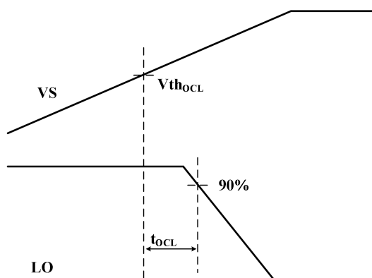
图3 V_s > V_{th_{OCL}} 至输出关断的波形及参数定义
