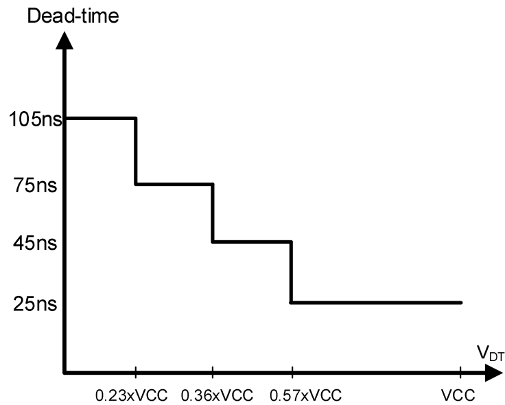
图7-8 MSA2092 中死区时间与 V_{DT} 的关系
