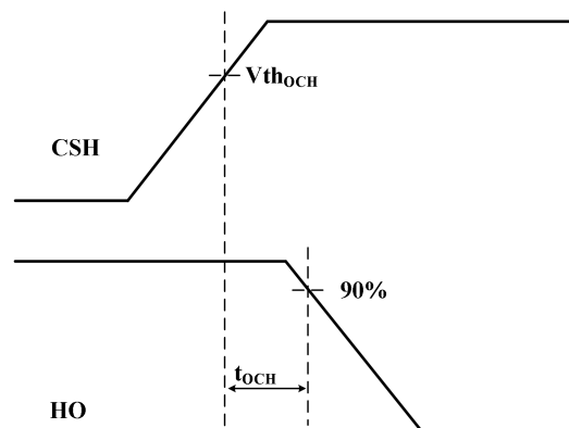
图4 V_{CSH} > V_{th_{OCH}} 至输出关断的波形及参数定义
