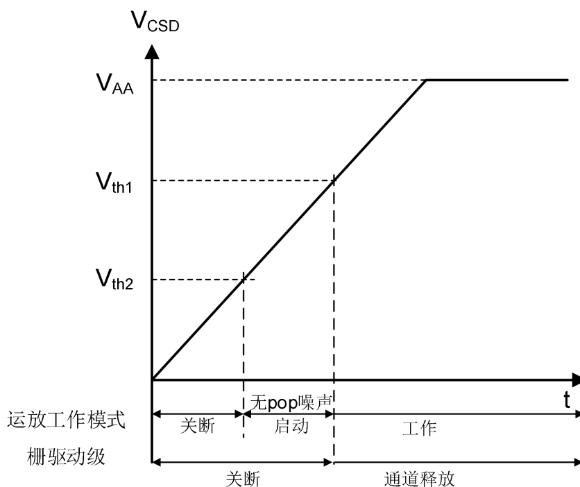
图 7-5 MSA2092 VCSD 和运算放大器的工作模式
