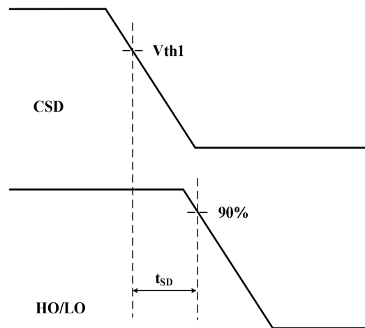
图2 CSD信号至输出信号关断波形及参数定义
