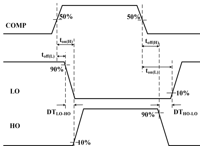
图1 开关波形及参数定义
