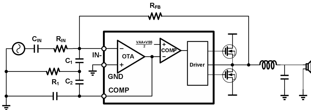
图7-3 MSA2092 典型控制环路设计
