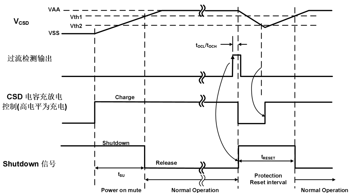
图 7-6 过流保护时序图
