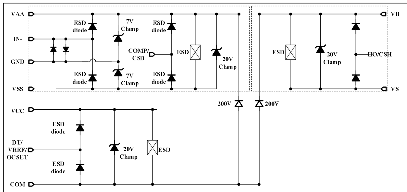
芯片I/O 端口等效电路图
