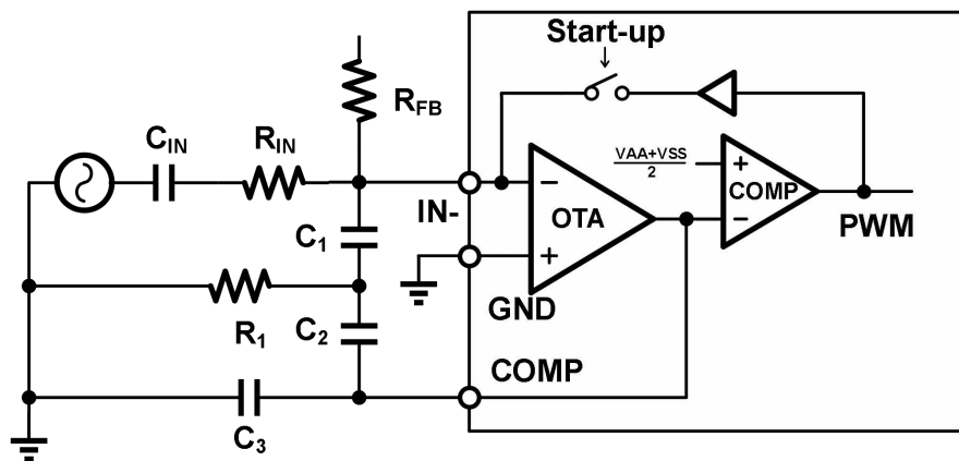
图 7-4 MSA2092 “咔哒”噪声消除机制
