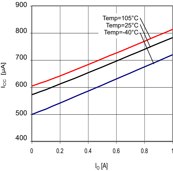
Fig.30 I_o-I_{cc}
