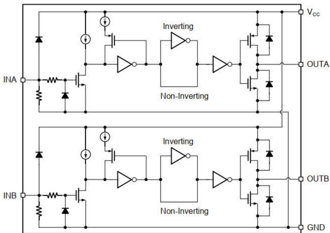
图 8-1 IRS4427/IRS4427S 功能框图
