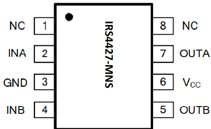
图5-1 8-脚 SOIC-8/PDIP-8 顶视图
