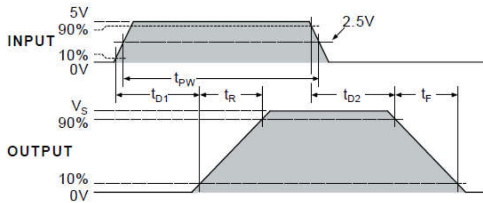
图 7-1 输入输出(同相)波形图
