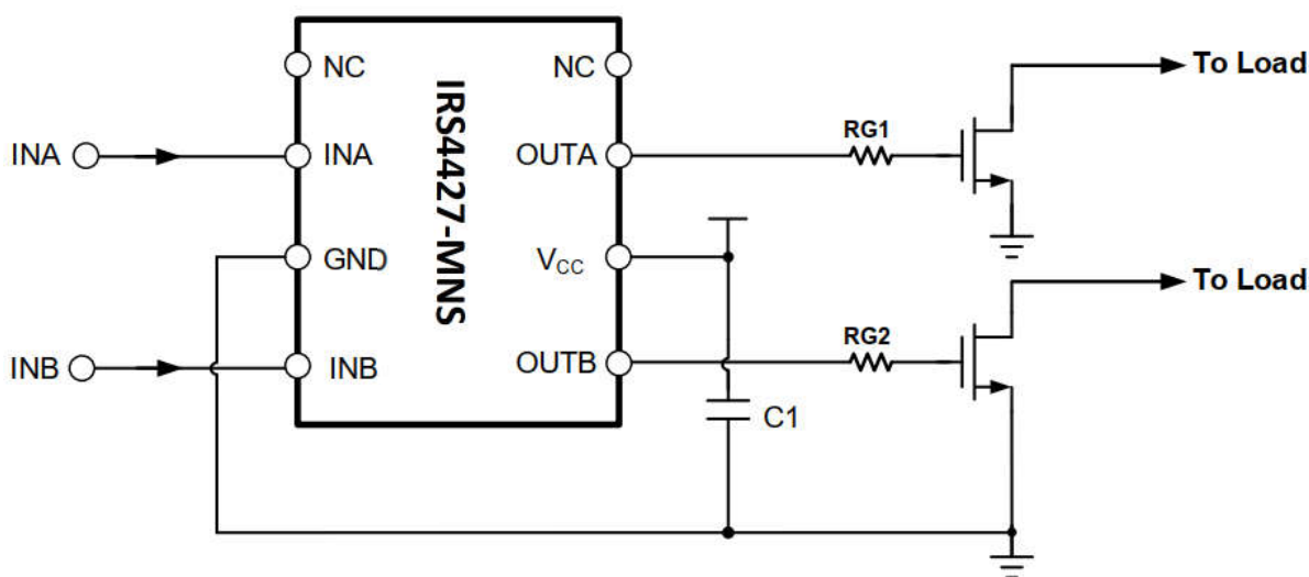
图 9-1 IRS4427/IRS4427S 典型应用电路图
