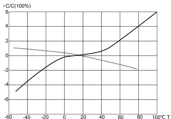
容量与温度曲线图
