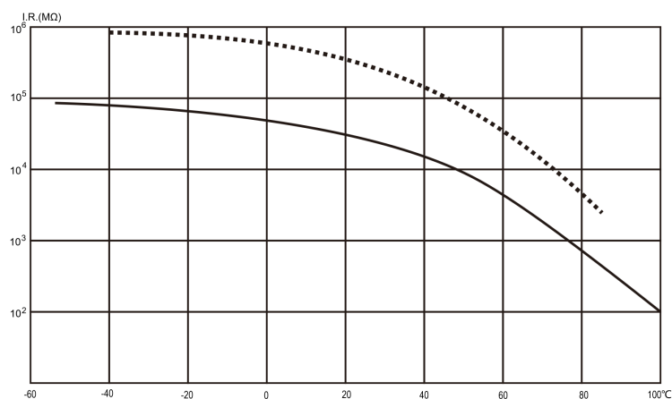
绝缘电阻与温度曲线图
