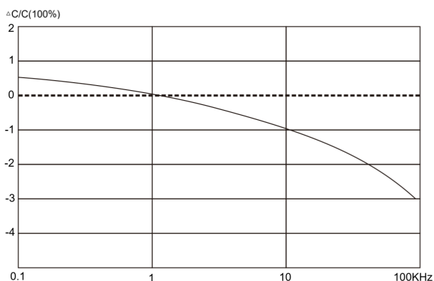
容量与频率曲线图
