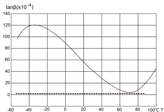
损耗角正切与温度曲线图
