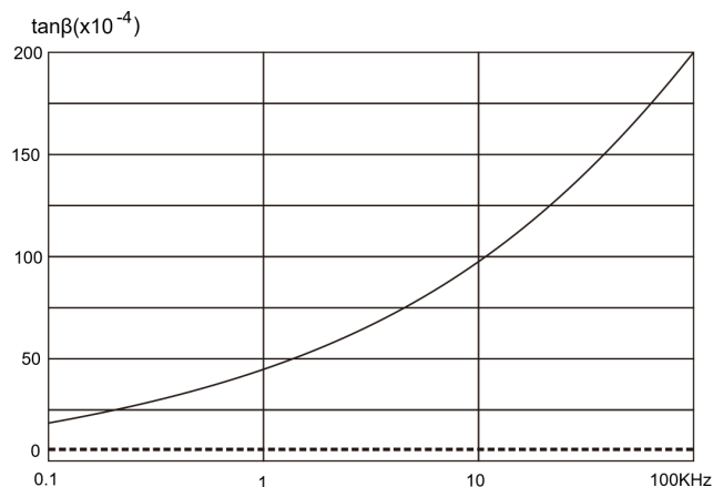
损耗角正切与频率曲线图
