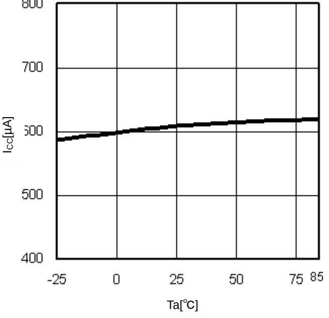
Fig.10 T_a-I_{cc}
