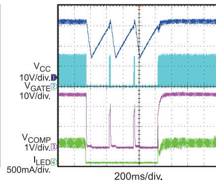
OVP
