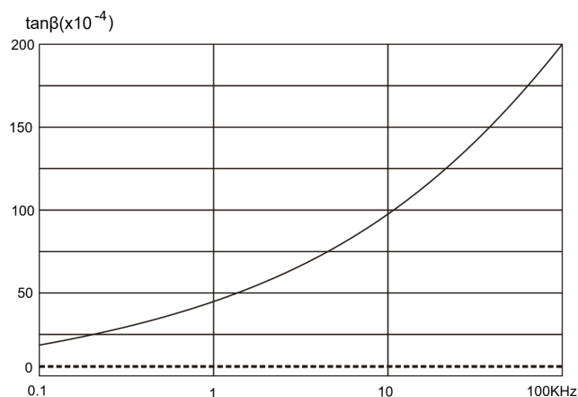
损耗角正切与频率曲线图
