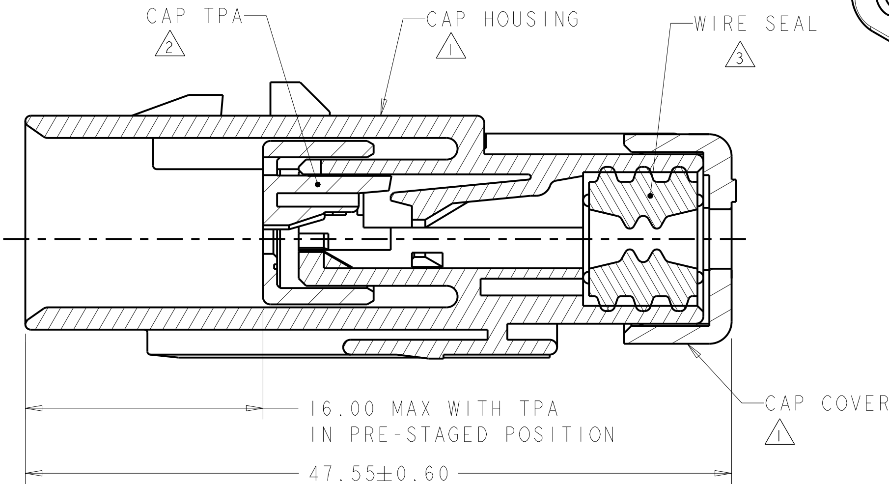
SECTION A-A
