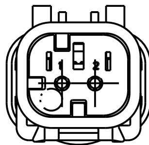
2320913-3 SCALE 2:1 KEY C
