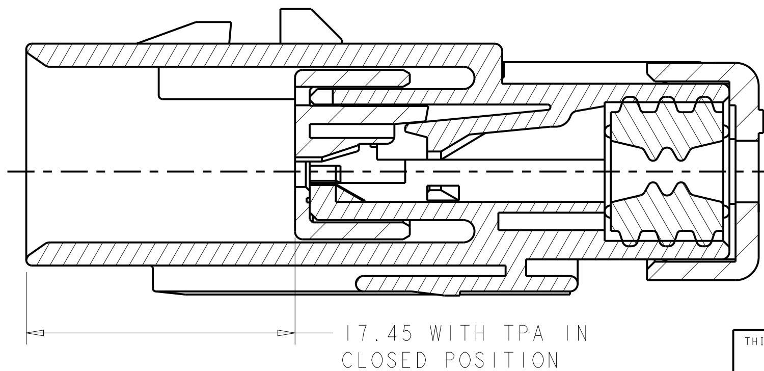
SECTION A-A
