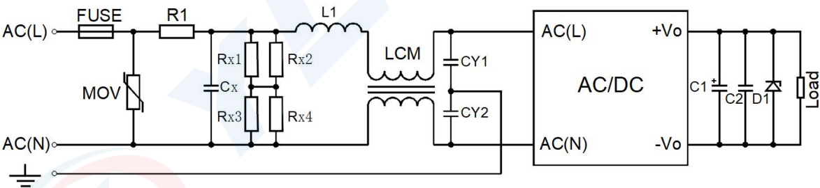
EMC 解决电路推荐参数值
