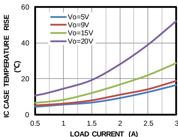
Thermal Rise
