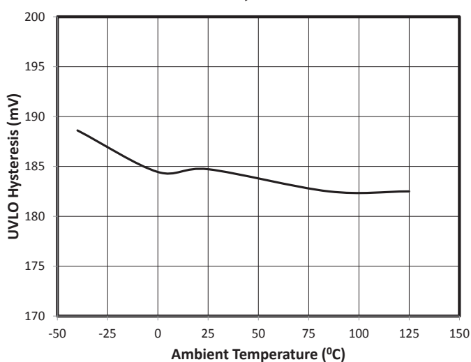
UVLO Hysteresis
