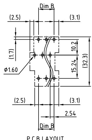
P.C.B LAYOUT
