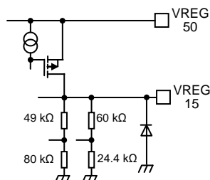
2) VREG15 pin
