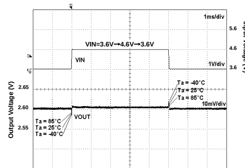
Fig 154. VIN Response
