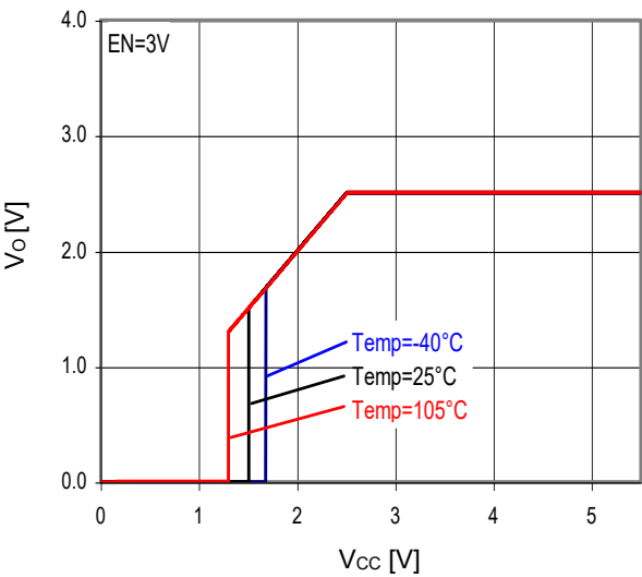
Fig.27 V_{cc}-V_o ( I_o=0\text{mA} )
