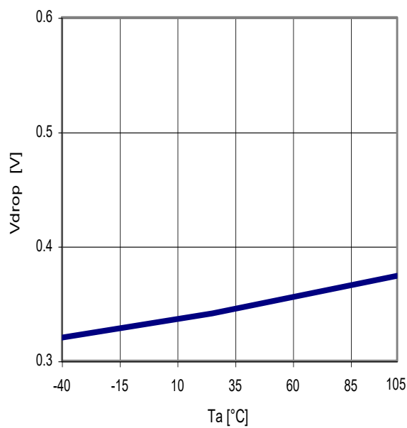
Fig.33 T_a - V_{drop} V_{cc}=3.3\text{V} , I_o=0.5\text{A}
