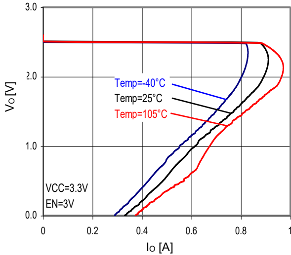
Fig.29 OCP
