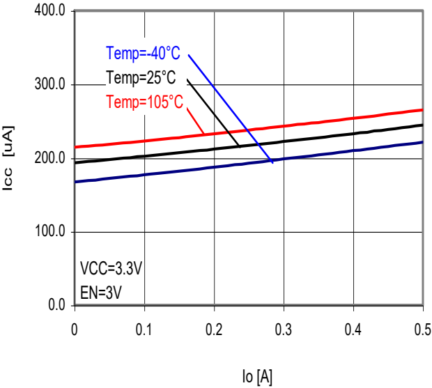
Fig.30 I_o-I_{cc}
