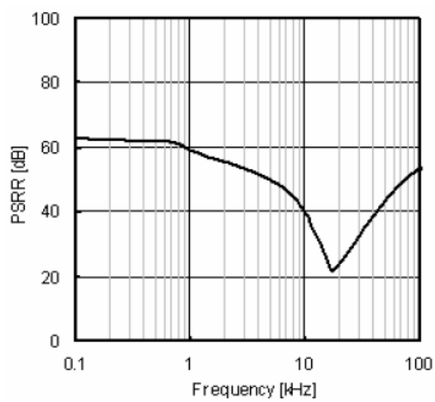
Fig.32 PSRR ( I_o=0\text{mA} )
