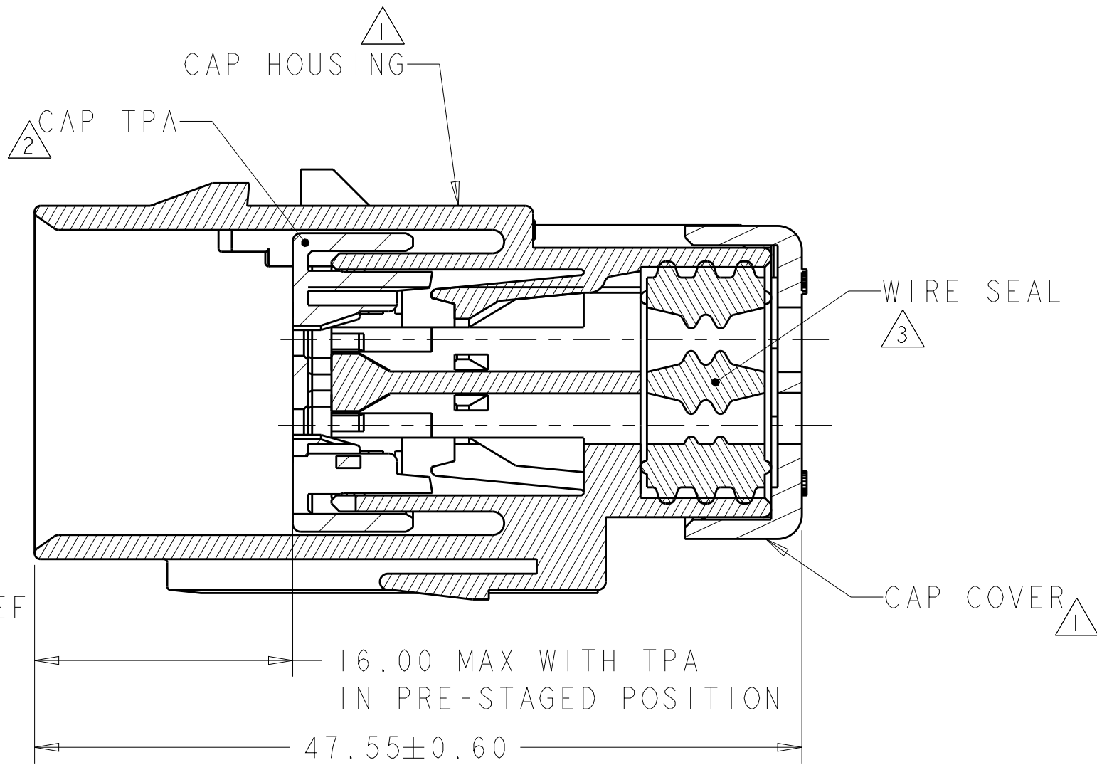
SECTION A-A
