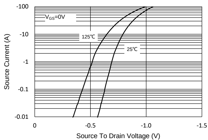
Fig.9 - I_S - V_{SD}
